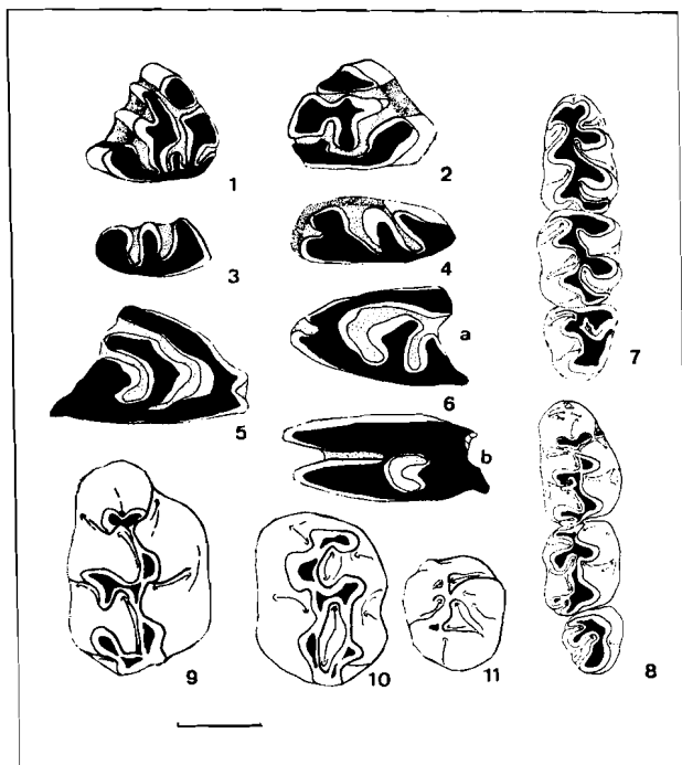
FIG. 3. — Prolagus oeningensis KONIG 1825, de Escobosa; 1: P/3 izq., Es-3. 3: P2/dcho., M-1021. 5: P3/dcho., M-1022. Prolagus tobiensis LÓPEZ nov. sp. de Escobosa; 2: P/3 dcho., Es. I-1, holotipo. 4: P2/izq., M-1001. 6 a y b: P3/-P4/izq. en conexión, M-1002. Megacricetodon crusafonti FREUDENTHAL 1963, de Escobosa; 7: Serie dentaria inf. izq., M-2507. 8: Serie dentaria sup. dcha., M-1508. Cricetodon aguirrei SESE nov. sp.; 9: M1/dcho., M-167. 10: M2/izq., M-216. 11: M3/izq., M-106.
