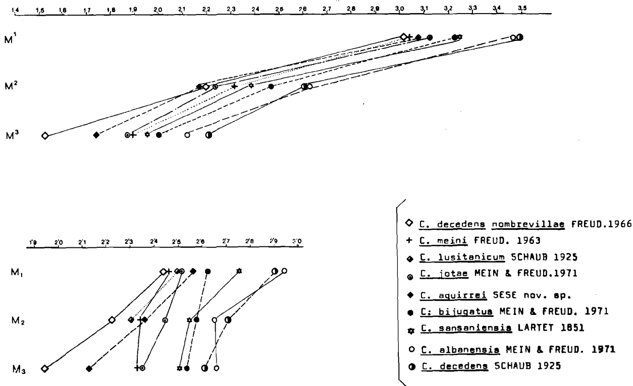
FIG. 2. — Gráfico de la longitud media de los molares superiores e inferiores de varias especies del género Cricetodon . Medidas tomadas en BAUDELOT 1972, FREUDENTHAL 1963 y 1966, MEIN & FREUDENTHAL 1971, a y b) y SCHALB 1925.
