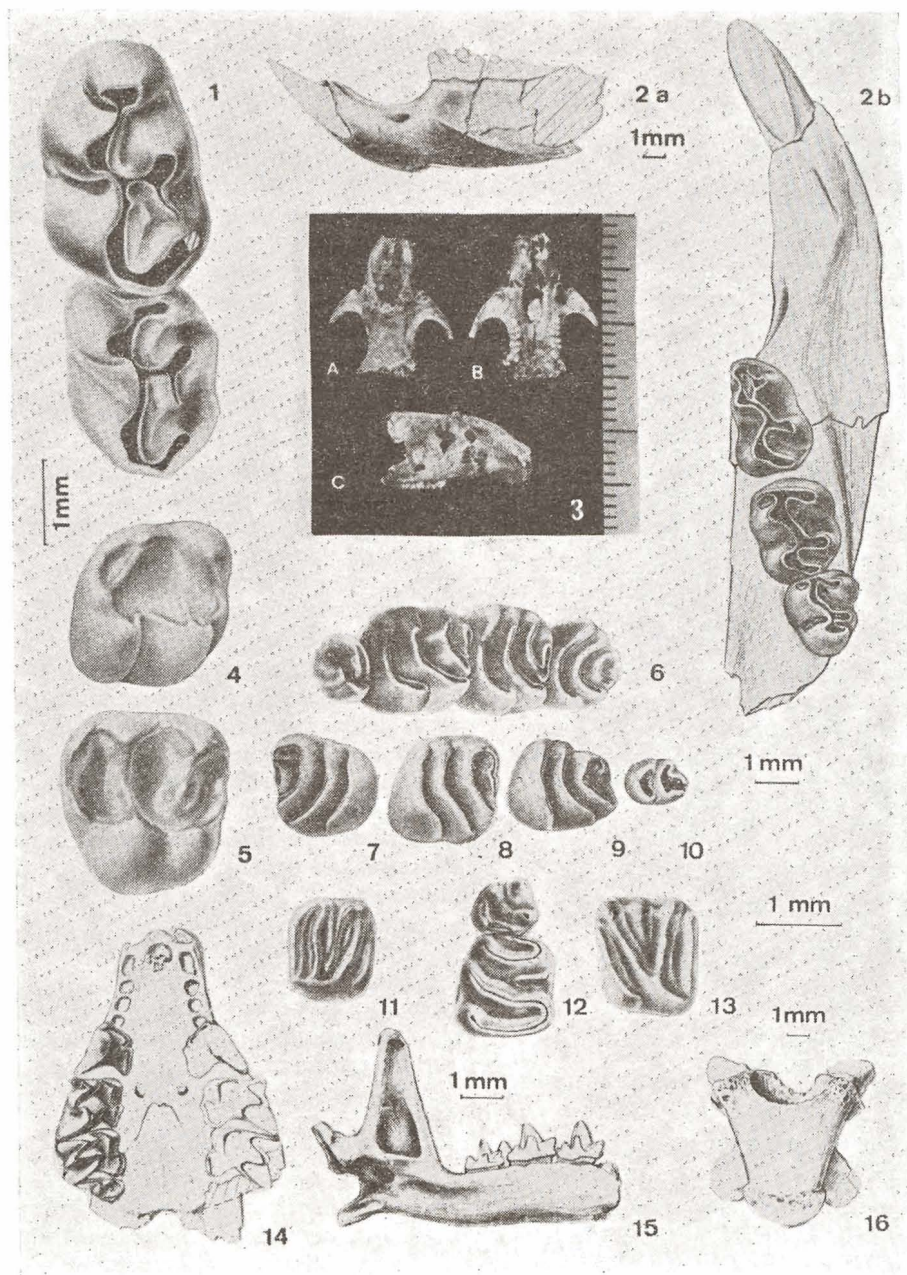
FIG. 4. — Cricetodon aguirrei SESE nov. sp. (Fig. 1: Holotipo: M1/-M2/izq., Es. 221-224.) (Fig. 2: Paratipo. Mandíbula izq., M-001: a = vista lateral externa, b = vista oclusal.) — Megacricetodon crusafonto FREUDENTHAL 1963. (Fig. 3: Cráneo M-1602: a = vista superior, b = vista inferior y c = vista lateral.) — Heteroxerus grivensis (F. MAJOR 1909). (Fig. 4: M/1 inf. dcho., Es. 345.) (Fig. 5: M1/sup. dcho., Es. 398.) — Armantomys tricristatus LÓPEZ nov. sp. (Fig. 6: Holotipo. Maxilar sup. con P4/-M1/-M2/-M3/izq., M-1501.) (Fig. 7: Paratipo. M/3 izq., G/2-111.) (Fig. 8: Paratipo: M/2 dcho., M-70.) (Fig. 9: Paratipo. M/ dcho., M-77.) (Fig. 10: Paratipo. P/4 dcho., G/2-112.) — cf. Peridyromys dehmi DE BRUIJN 1966. (Fig. 11: M1-2/dcho., G/2-145.) — " Eliomys " cf. hartenbergi . (Fig. 12: P/4-M/1 izq., G/2-234.) (Fig. 13: M1-2/izq., G/2-233.) — Soricidae II. (Fig. 14: Cráneo M-1208, vista ventral.) (Fig. 15: Mandíbula G/2-2209, vista lateral interna.) — Gerrohontinae: Ophisaurus sp. (Fig. 16: Vértebra torácica.)
